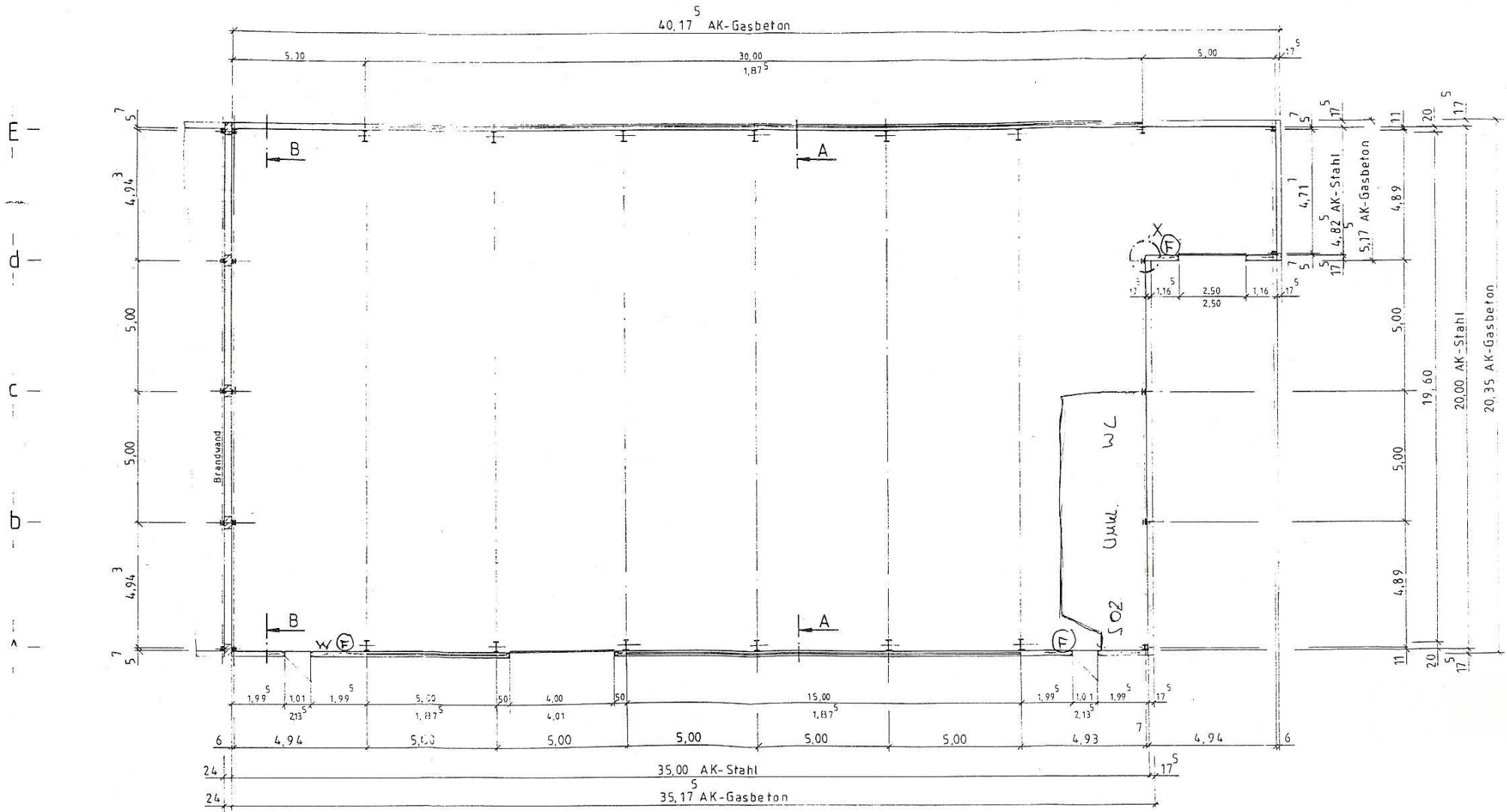
Grundriß
